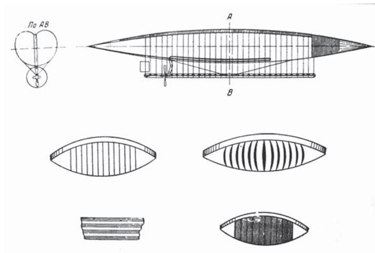
Рисунок Циолковского к работе «Теория и опыт аэростата, имеющего в горизонтальном направлении удлиненную форму».
