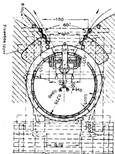
Схема пулеметного ДОТа легкого типа
