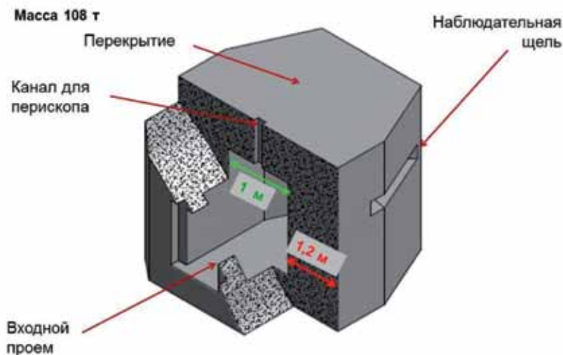
Схема Монолитного командирского наблюдательного пункта с тремя смотровыми щелями
