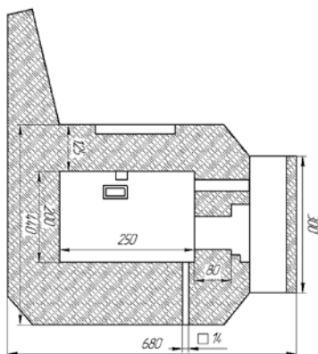
Схема ДОТ № 5, Чертеж ВПО «Ильинский патруль», 2016 год
