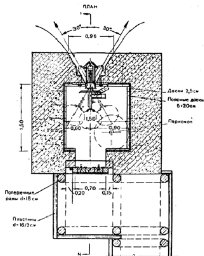
Схема ДОТа «Наставление по полевой фортификации РККА», 1943 год
