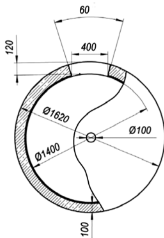
Схема пулеметного ДОТа легкого типа
