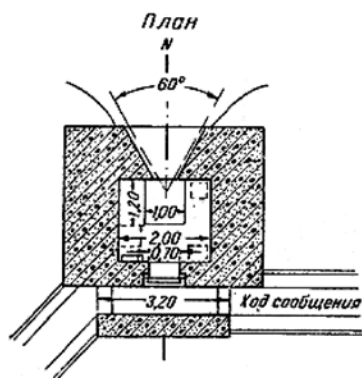
Схема ДОТа «Наставление по полевой фортификации РККА», 1939 год
