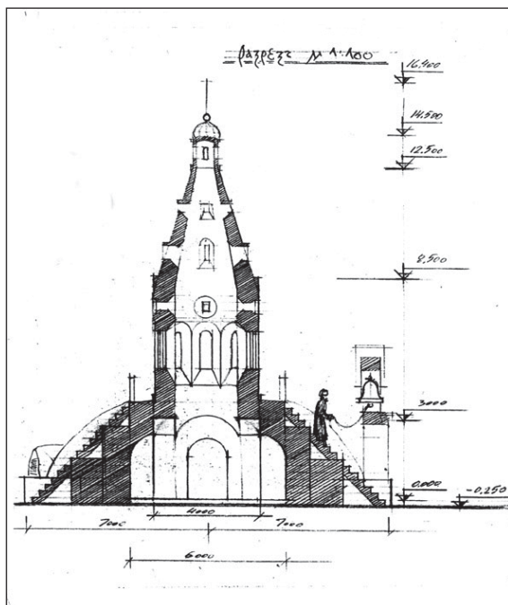
Эскизный проект памятника-часовни. Автор проекта Д. Власов
