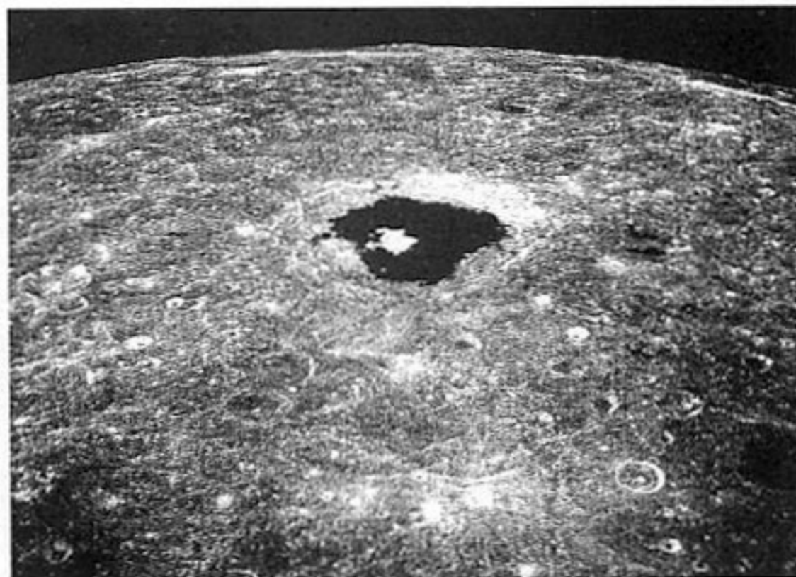
Кратер «Циолковский», снятый экипажем космического корабля «Аполлон-15»
