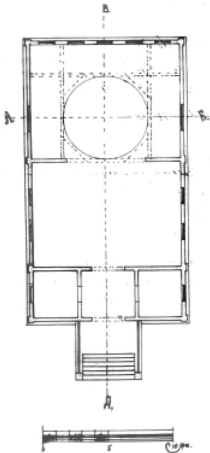
ПЛАНЪ.
