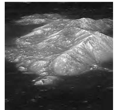
Центральная горка кратера Циолковский, снятая космическим аппаратом LRO в ноябре 2013 года (вид с запада на восток). Ширина снимка около 25 км
